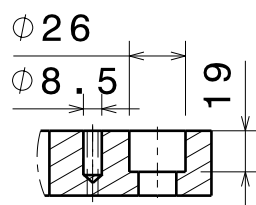
Détail C
